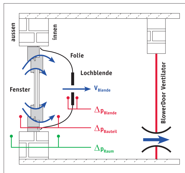
Prinzipische Darstellung zur Bestimmung der Fugendurchlässigkeit von Fenstern
